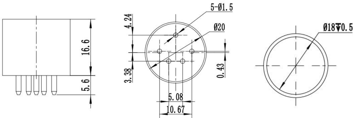
图 2： 产品尺寸图
